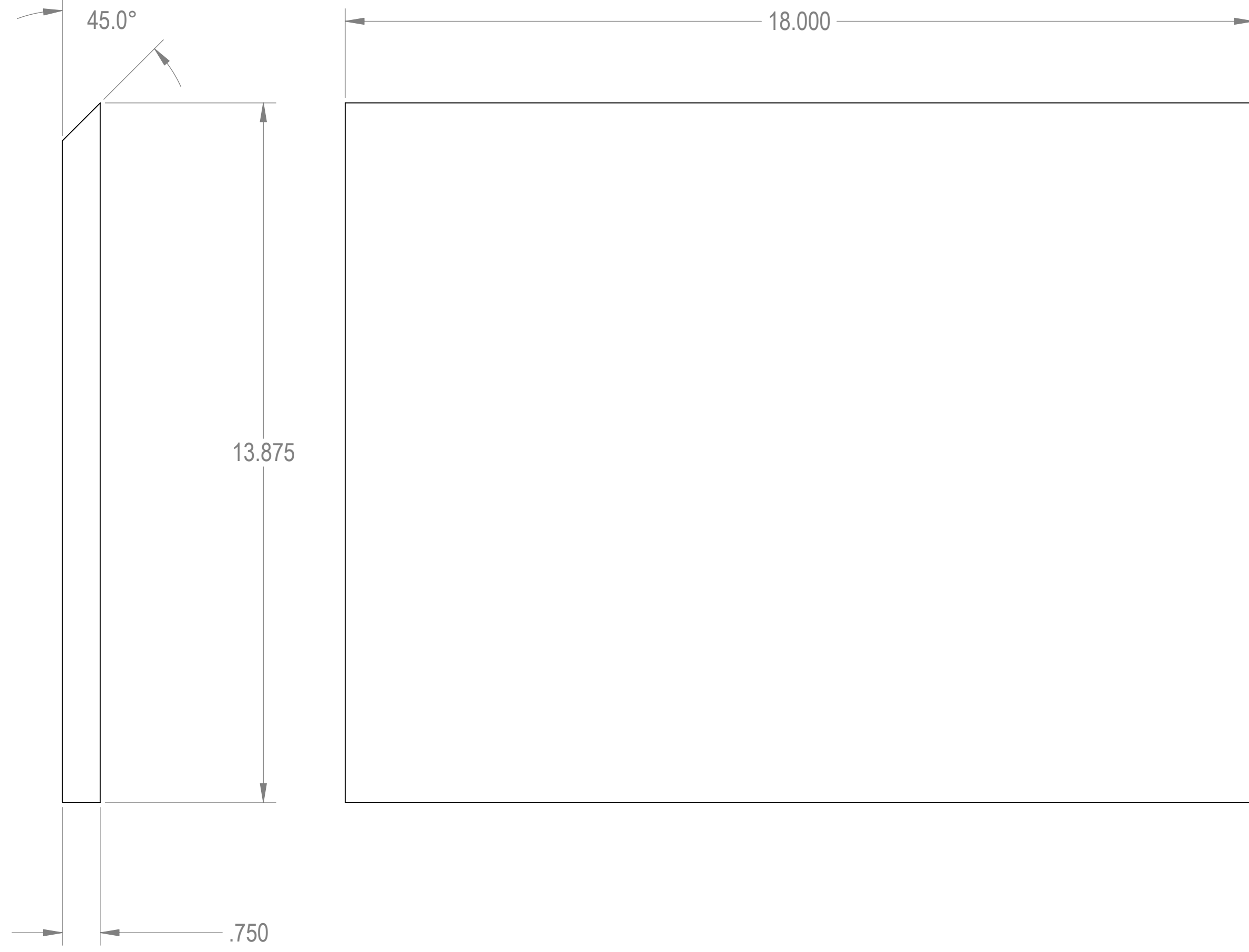
BOX DOOR
